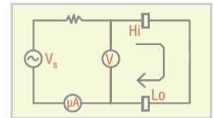
回路短絡時： C_m \gg C_x
