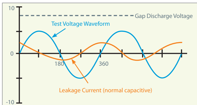
圖 1: 正常波形
