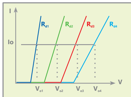
図2：数の異なるLEDシミュレーション
