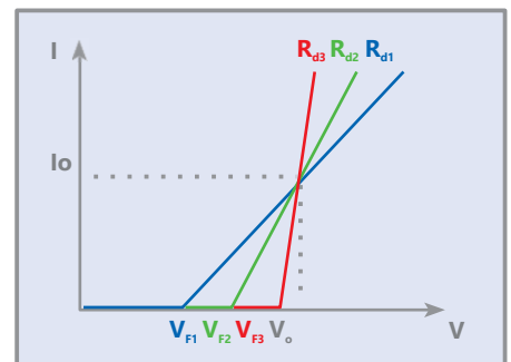
図3：特性の異なるLEDシミュレーション
