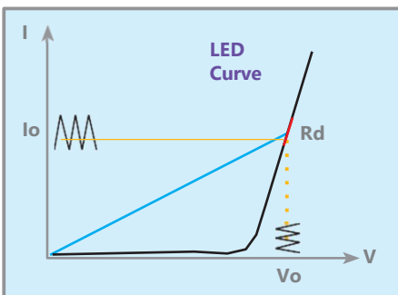
図1：LED V-I曲線（特性）
