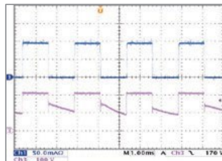
図5：LEDロードシミュレータ調光電流波形
