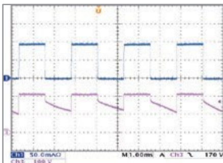
図4：LED実負荷調光電流波形
