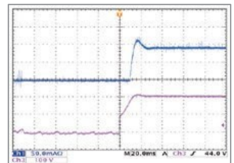
図6：LED電源ドライバーターンオン時の波形
