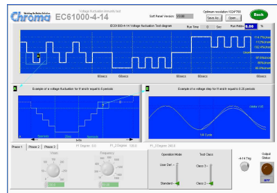
IEC 61000-4-14 電圧変動イミュニティ試験
