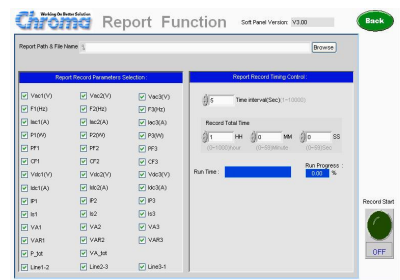
測定結果記録設定画面
