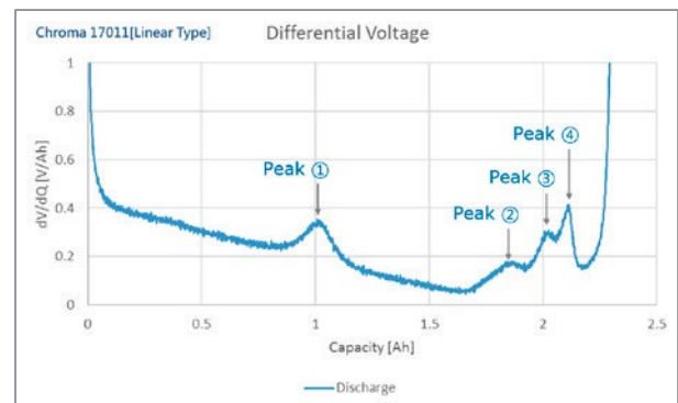
dV/dQ曲線
