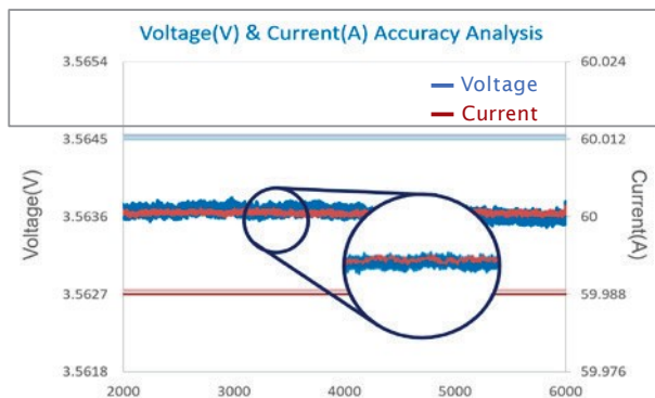
電圧・電流の実測定精度
