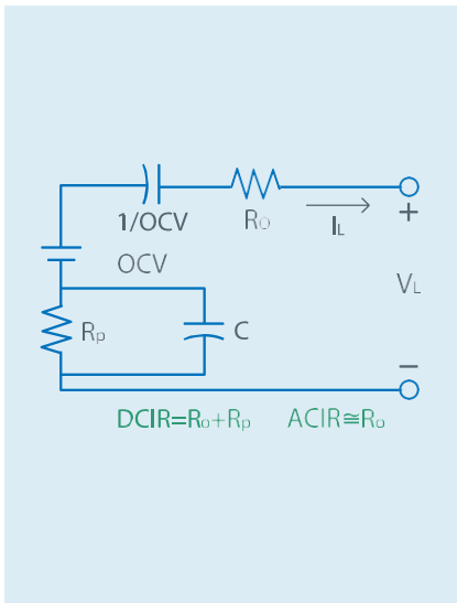
リチウムイオン電池 等価回路モデル
