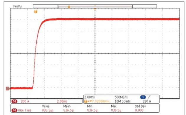
ハイブリッドパルスパワー特性 (HPPC)
