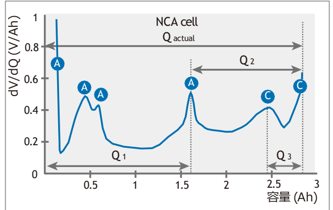
dV/dQ 曲線
