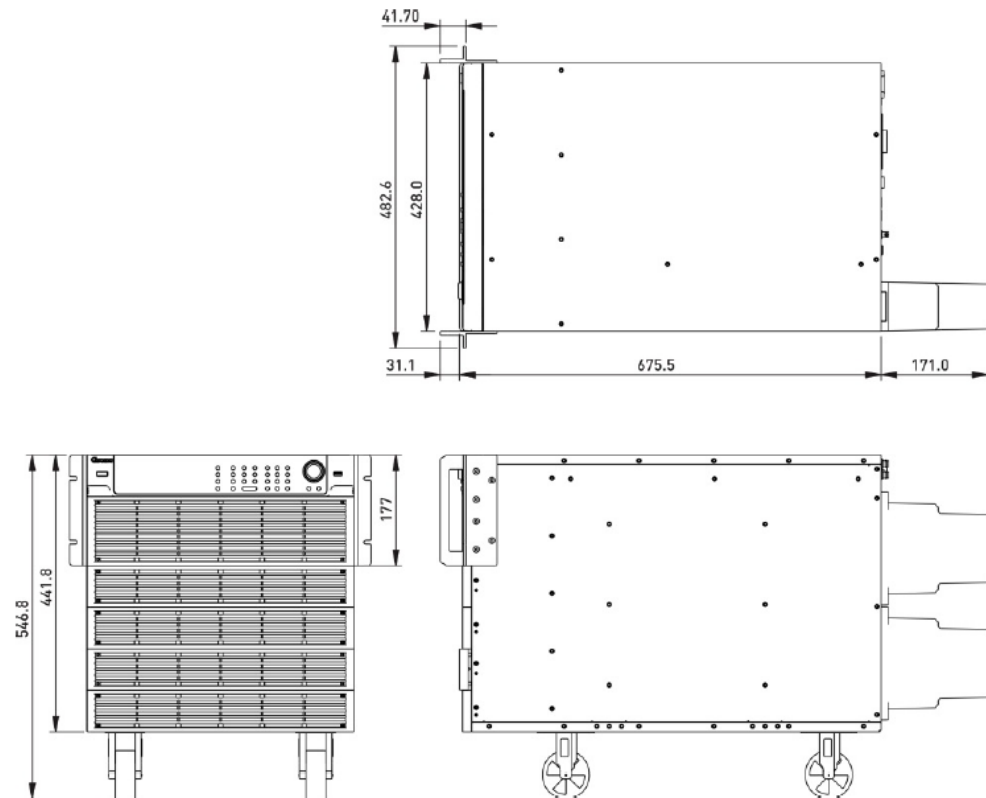
63215A/63218Aシリーズ外観
