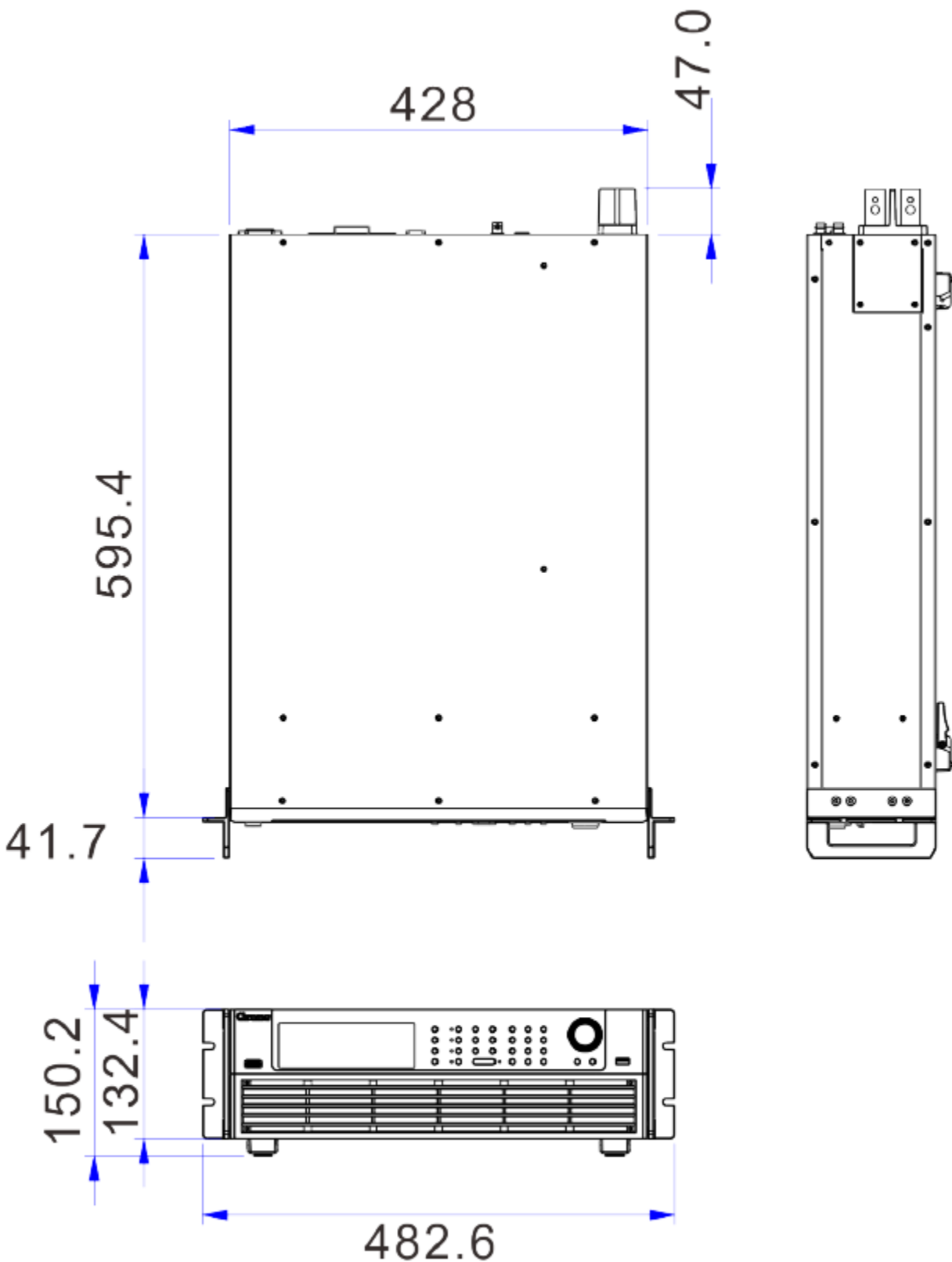
63202A/63203Aシリーズ外観 (端子カバー無)
