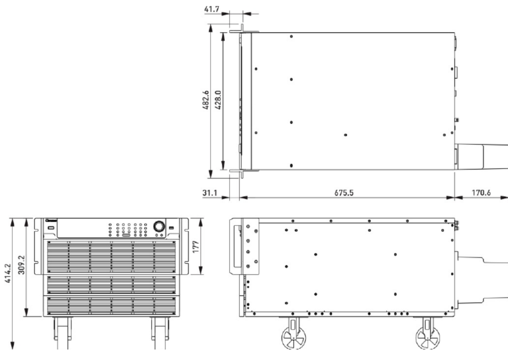
63208A/63210A/63212Aシリーズ外観
