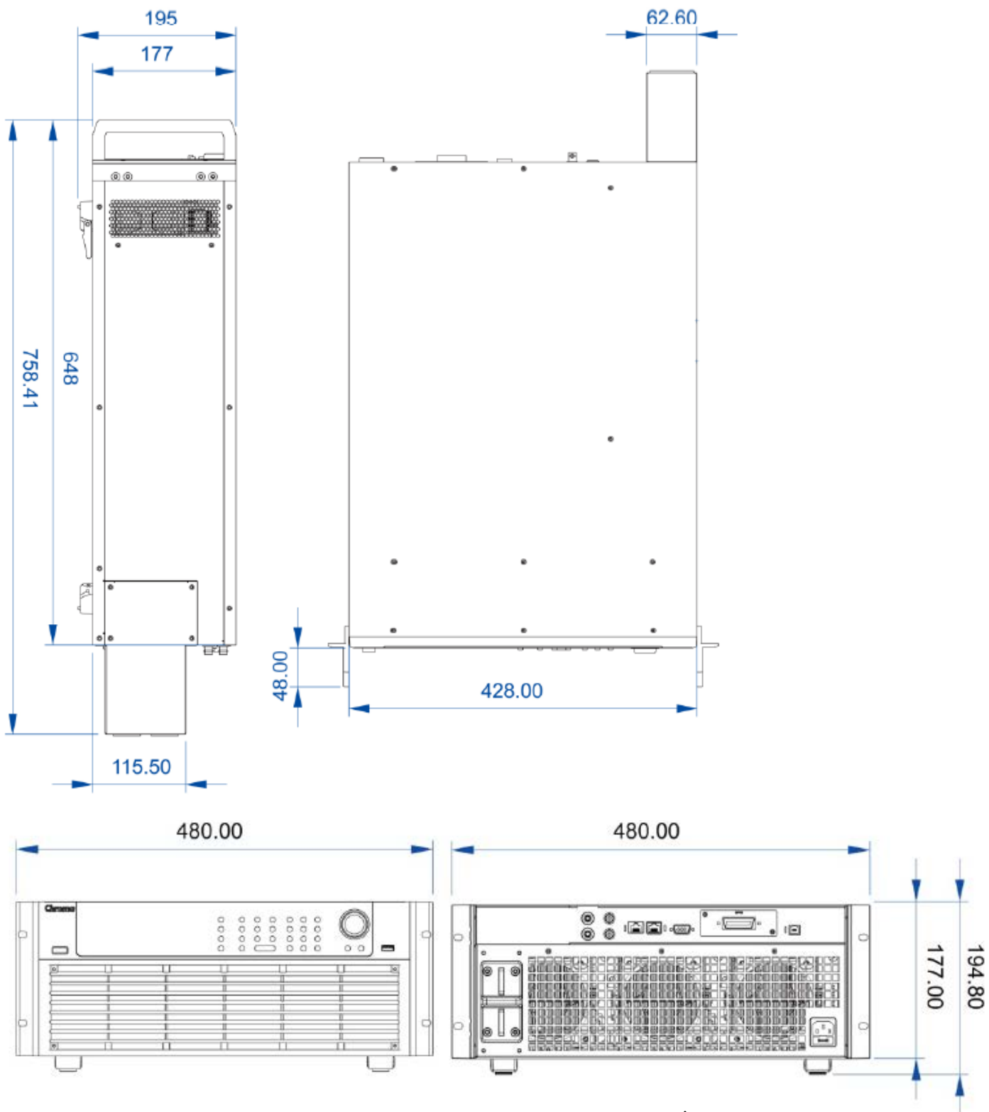
63204A/63205A/63206Aシリーズ外観
