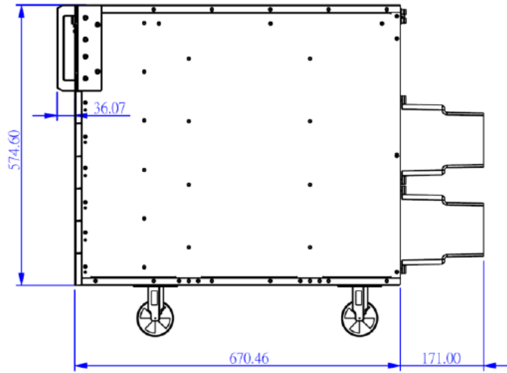
63220A/63224Aシリーズ外観
